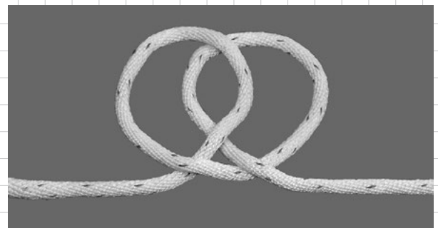
Mastwurf gelegt
