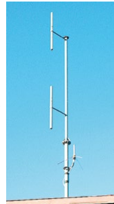
Relaisfunkstelle
